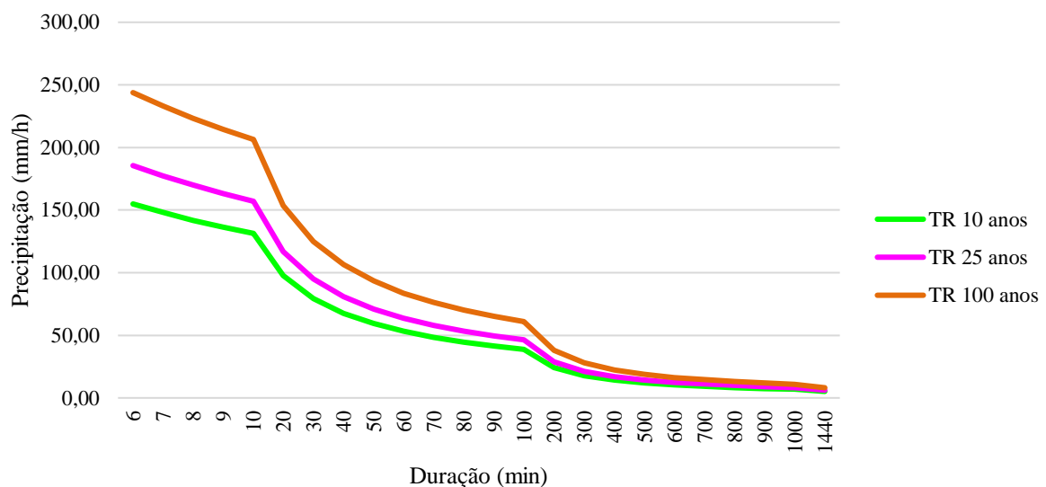
Figura 5 - Curva intensidade-duração-frequência.
